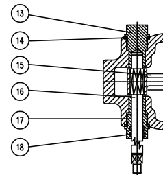
A-A Section
