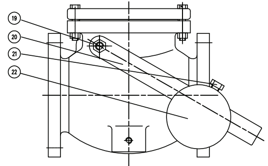
A-A Section
